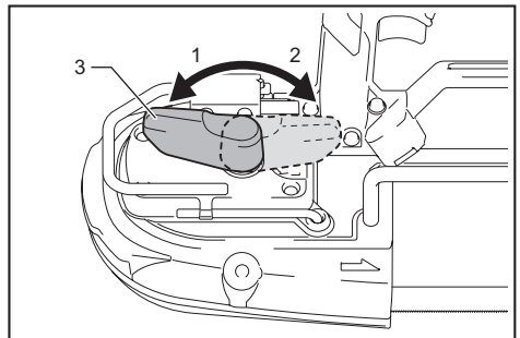
► 1. Serrer 2. Desserrer 3. Levier de serrage de la lame
